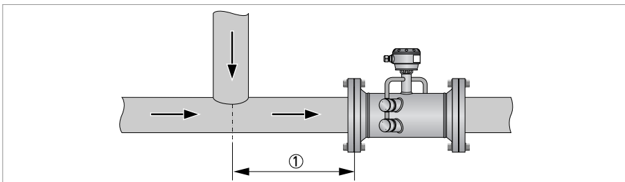
Рисунок 3-6: Расстояние после Т-образной секции
