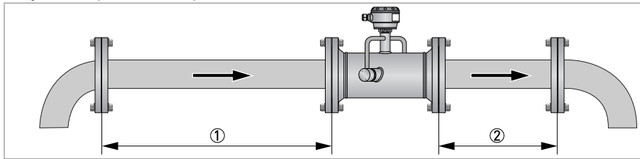
Рисунок 3-1: Рекомендуемые длины прямых участков на входе и выходе прибора для \leq DN80/3 дюйма
