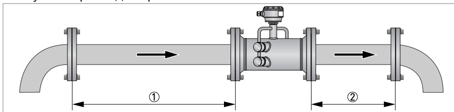
Рисунок 3-2: Рекомендуемые длины прямых участков на входе и выходе прибора для \geq DN100/4 дюйма
