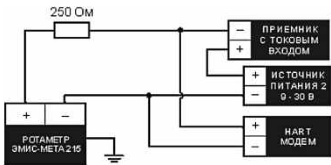
Рисунок 6. Схема подключения токового и цифрового выхода ротаметра
