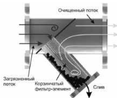
Рисунок 1. Устройство фильтров
