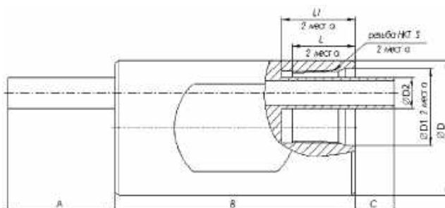
Рисунок 6. Габаритные и присоединительные размеры преобразователей
