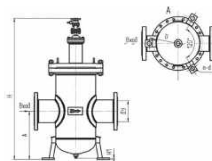
Рисунок 5. ЭМИС-ВЕКТА 1212 с креплением крышки по периметру (выше Ду > 50мм)
