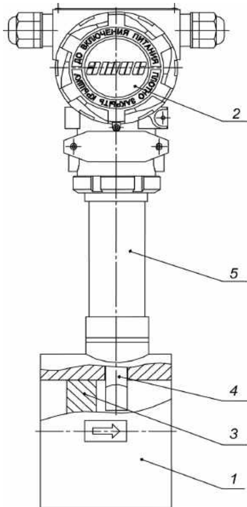
Рисунок 1. Устройство расходомера
