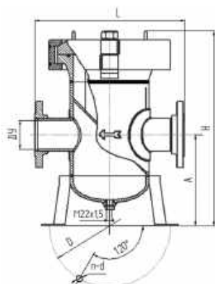
Рисунок 3. Габаритные и присоединительные размеры фильтров ЭМИС-ВЕКТА 1210 с быстрьюсъемной крышкой
