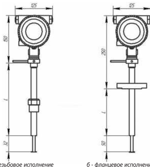
а - Резьбовое исполнение б - фланцевое исполнение Рисунок 5. Габаритные и присоединительные размеры расходомера
