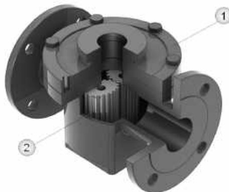
Рисунок 2. Конструкция первичного преобразователя
