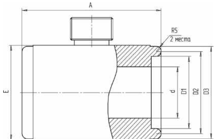
Рисунок 2. Устройство первичного преобразователя
