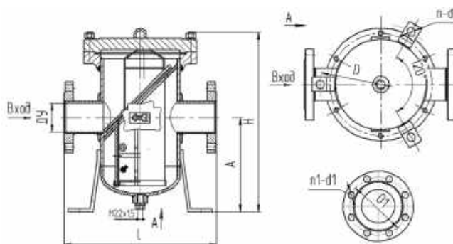
Рисунок 4. Габаритные и присоединительные размеры фильтров ЭМИС-ВЕКТА 1210 и с креплением крышки по периметру
