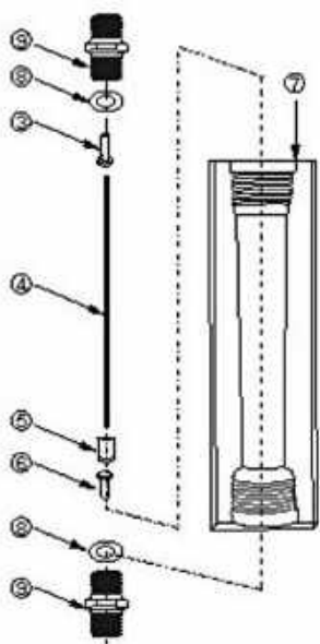
Рисунок 1. Устройство ЭМИС-МЕТА 210 проходной тип (ПР)
