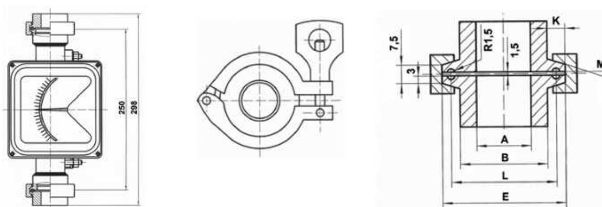
Рисунок 10. Присоединительные размеры приборов с зажимным соединением
