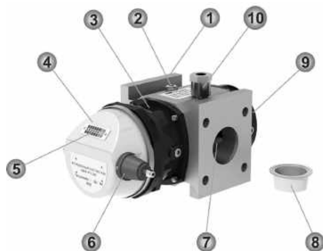
Рисунок 1. Устройство ЭМИС-РГС 245
